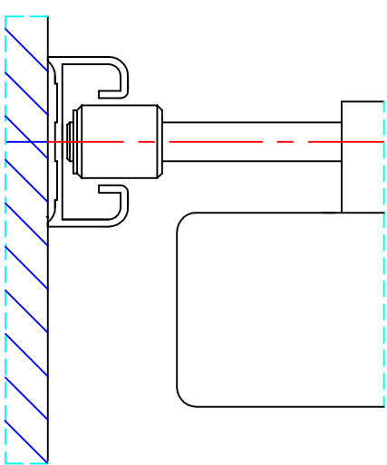
DETALLE INFERIOR
